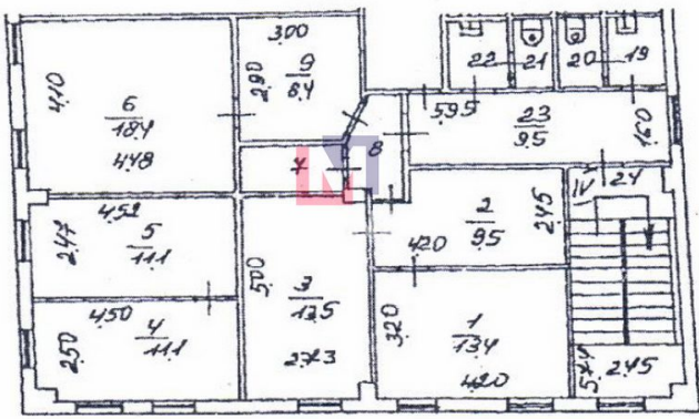
2 этаж
