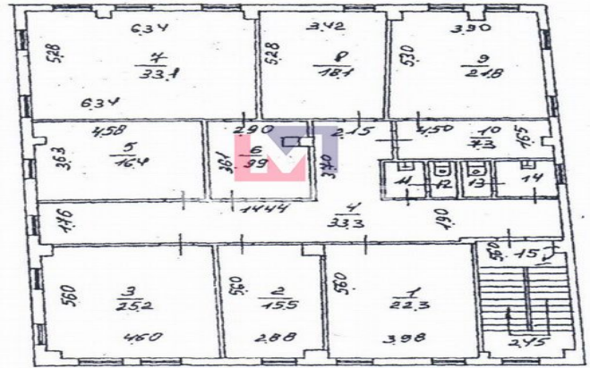
209 кв.м- 3 этаж
